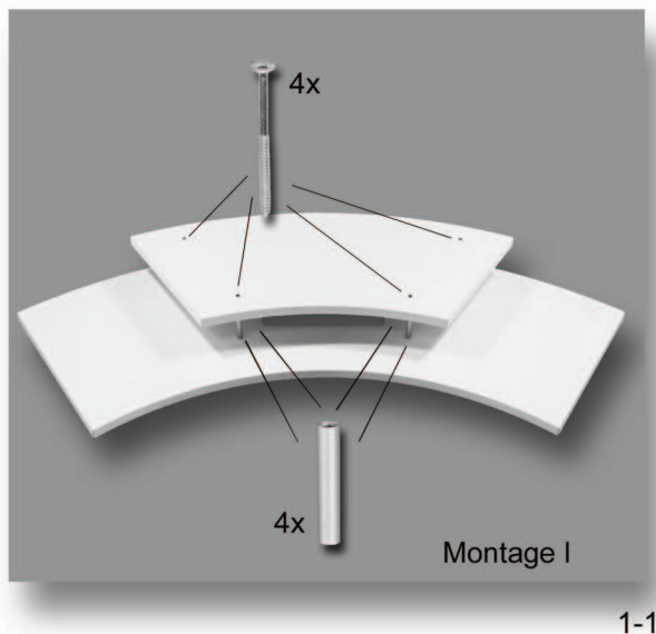
Montage Tischplatte „ohne“ Beleuchtung: 1
