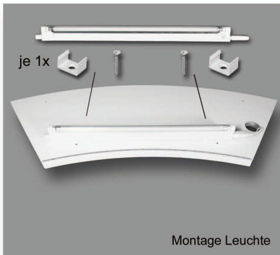
Montage Tischplatte „mit“ Beleuchtung
