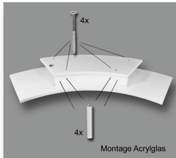
4x Hülse und 4x Schrauben leicht fixieren, Acrylglas einsetzen, Schrauben festziehen
